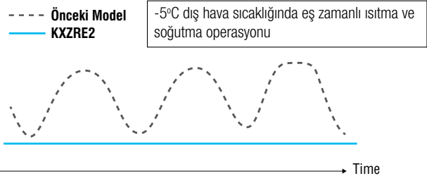
Soğutulan odada üfleme havası sıcaklıkları
